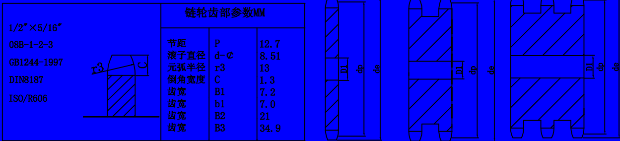
A型单排平片链轮
