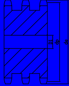
A型叁排平片链轮
