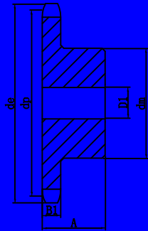
A型叁排平片链轮
